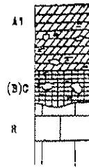
Rendzine brunifiée polycyclique
